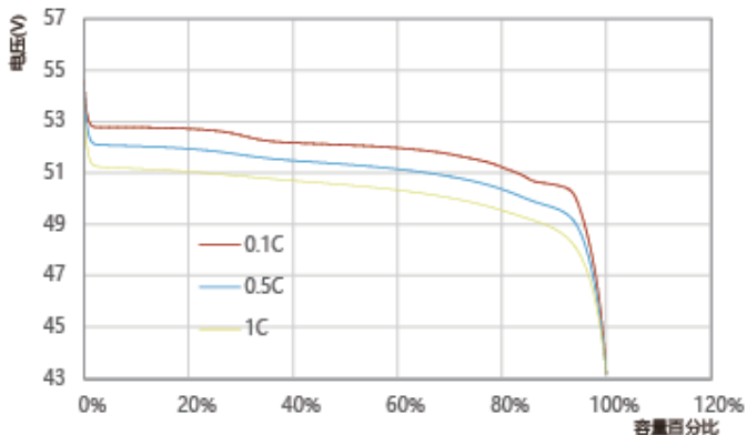
不同倍率下放电曲线 (25℃)
