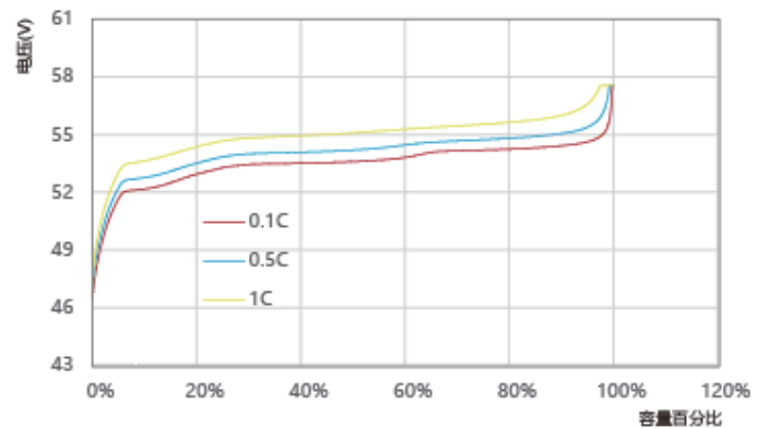
不同倍率下的充电曲线 (25℃)
