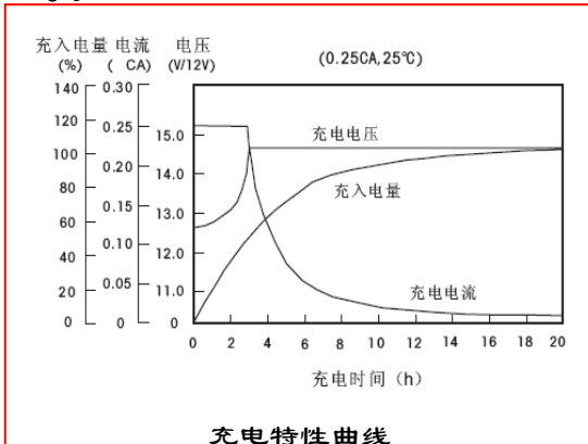
充电特性曲线
