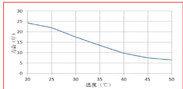
不同温度下浮充服务寿命曲线
